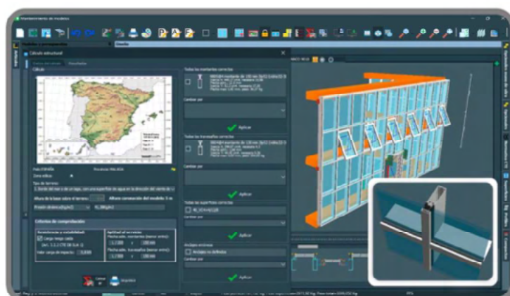
Vista de un muro cortina con tapeta y cálculo estructural
