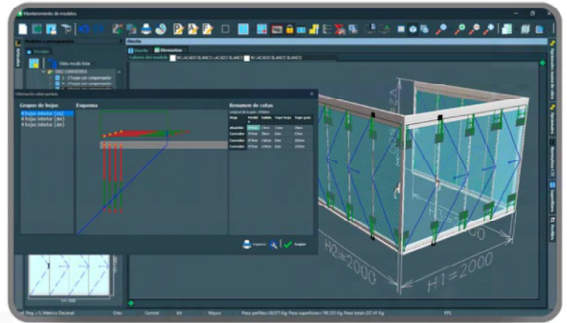
Esquema e información sobre apertura en modelos de cortina de cristal
